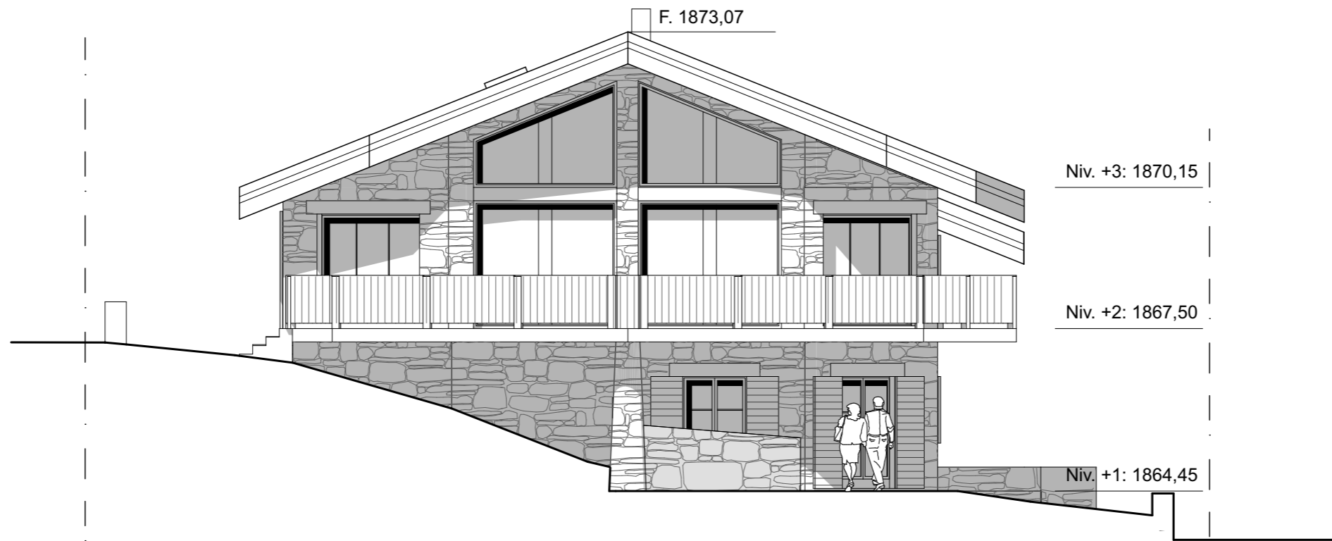
Façade SUD
